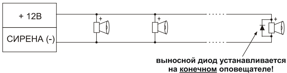
Рис. 6.2. Схема подключения нескольких звуковых оповещателей
