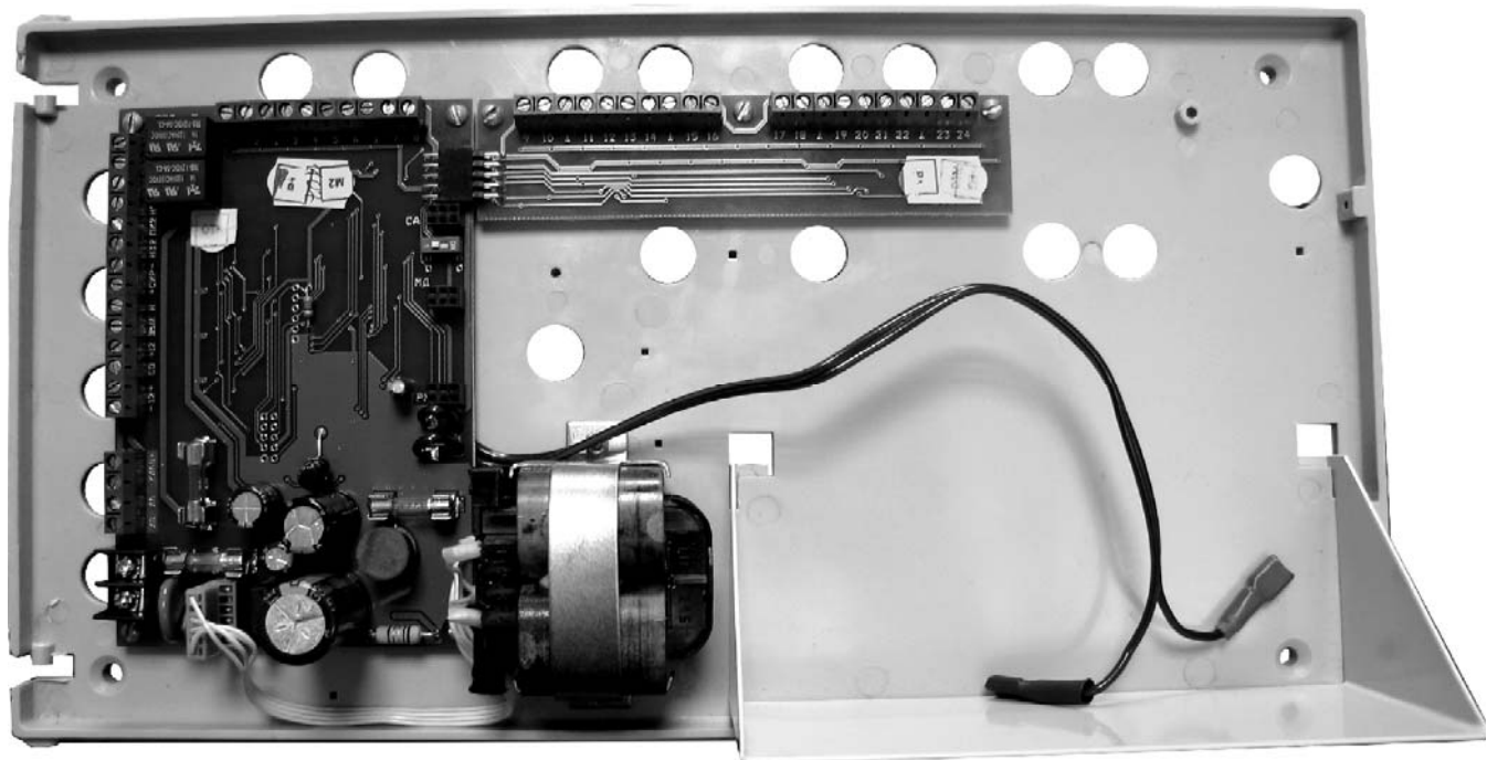
Рис.2. Устройство системного блока прибора со снятой крышкой
