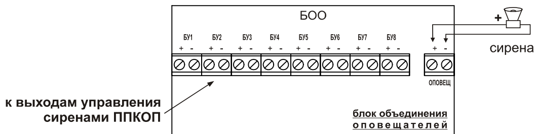
Рис. 6.3. Схема подключения одного звукового оповещателя (сирены) к нескольким приборам "Гранд МАГИСТР"
