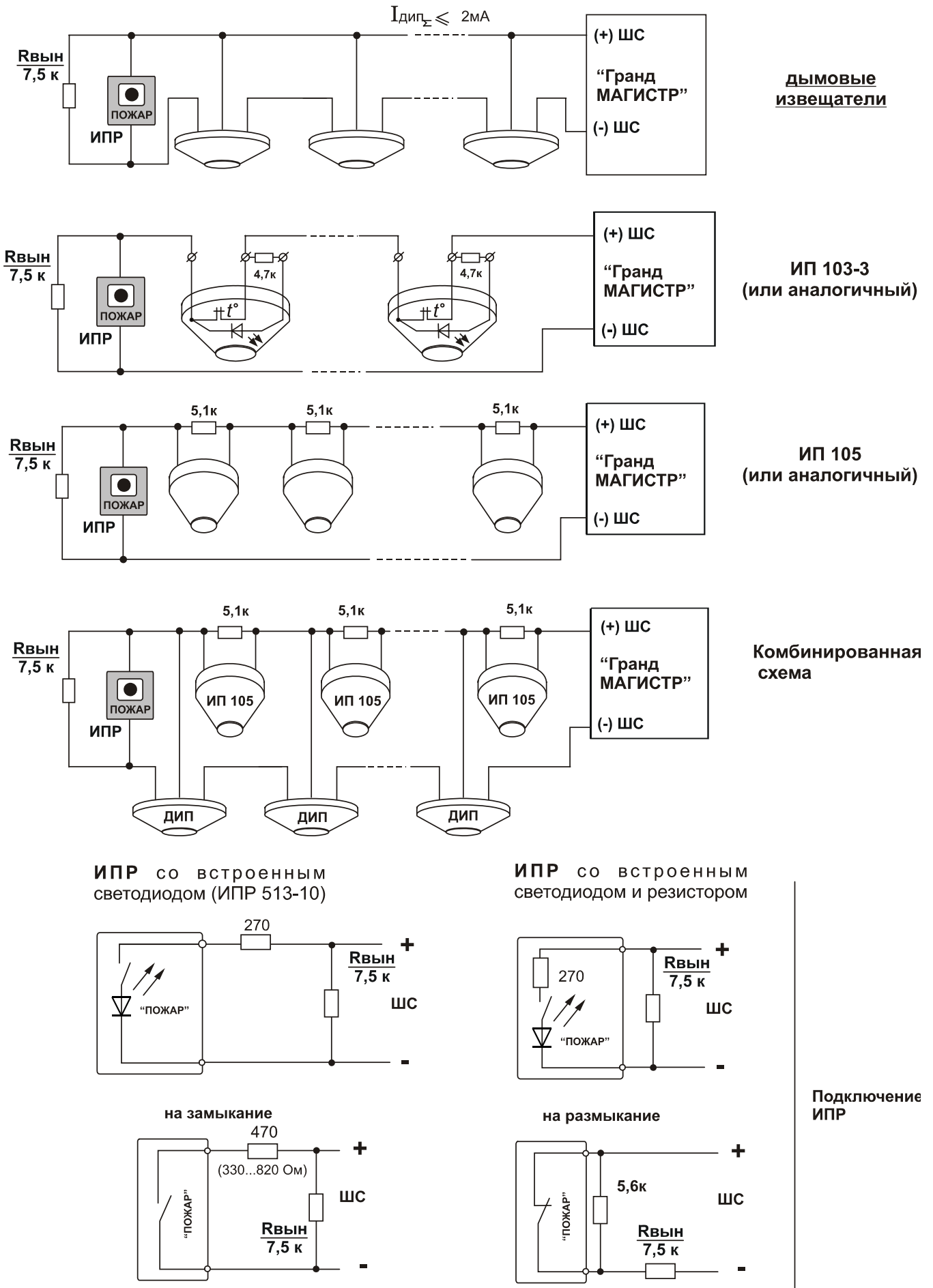
Рис. 4.3. Организация однопорогового шлейфа пожарной сигнализации
