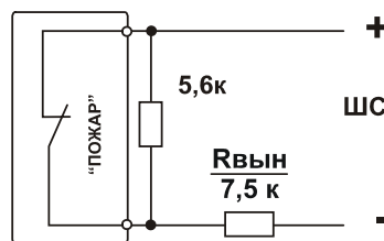
Рис. 4.2. Организация двухпорогового шлейфа пожарной сигнализации
