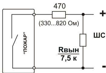
Рис. 4.2. Организация двухпорогового шлейфа пожарной сигнализации
